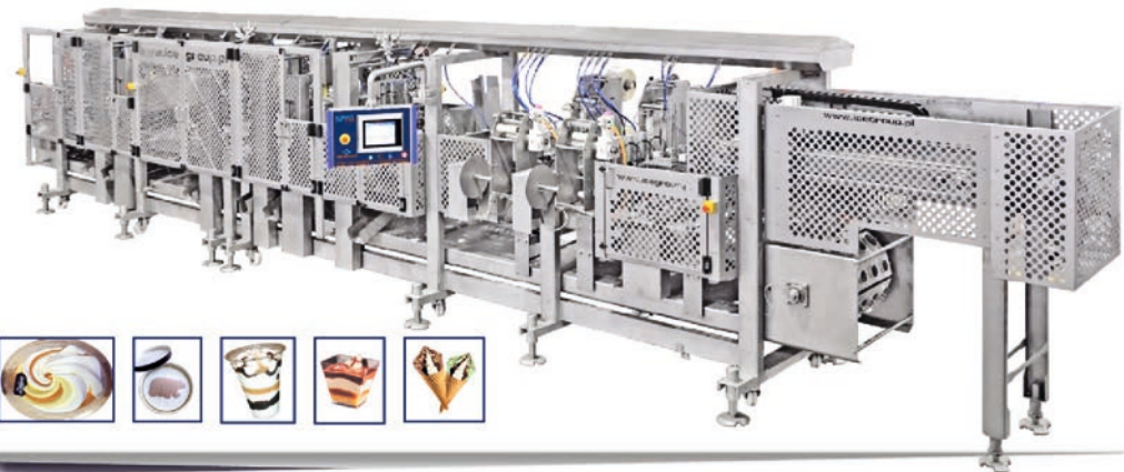
DESERTA LOG MACHINE
